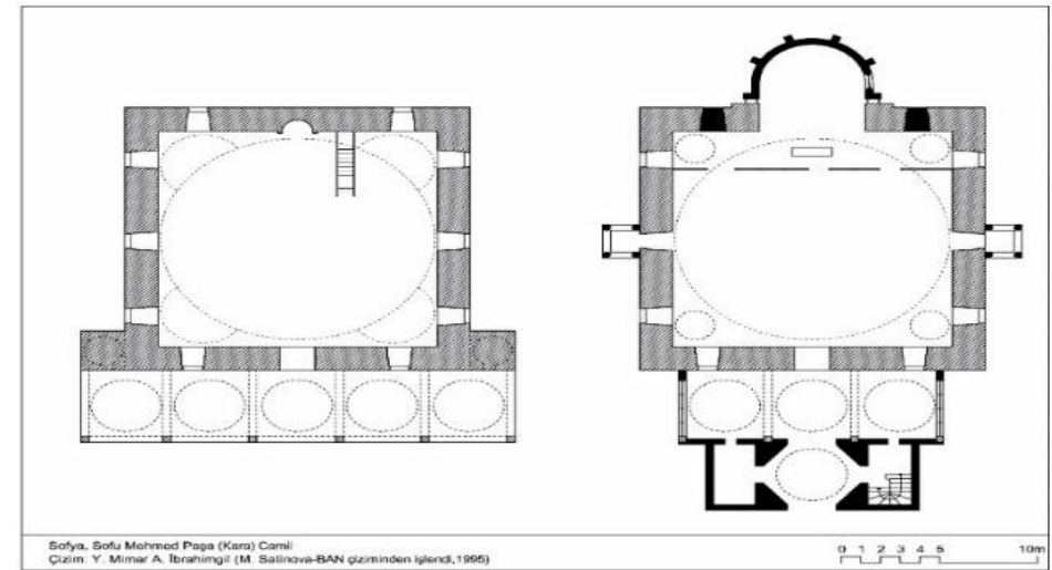
Sofya, Sofu Mehmed Paşa (Kara) Camii Çizim: Y. Mimar A. İbrahimî (M. Salinova-BAN çiziminden işlendi, 1995)
